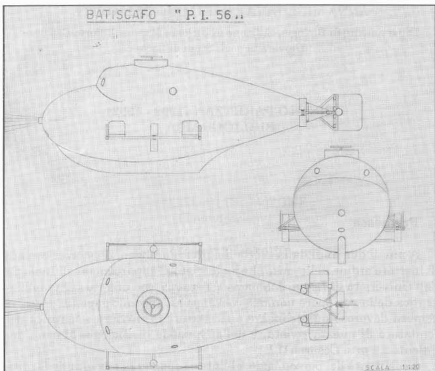
Fig. 1- Disegno originale (batiscafo P.I. 56) di una delle versioni dell' Ittioscafo che Pietro Parenzan aspirava di assegnare in dotazione alla comunità scientifica italiana, che ancora oggi ne è priva.
