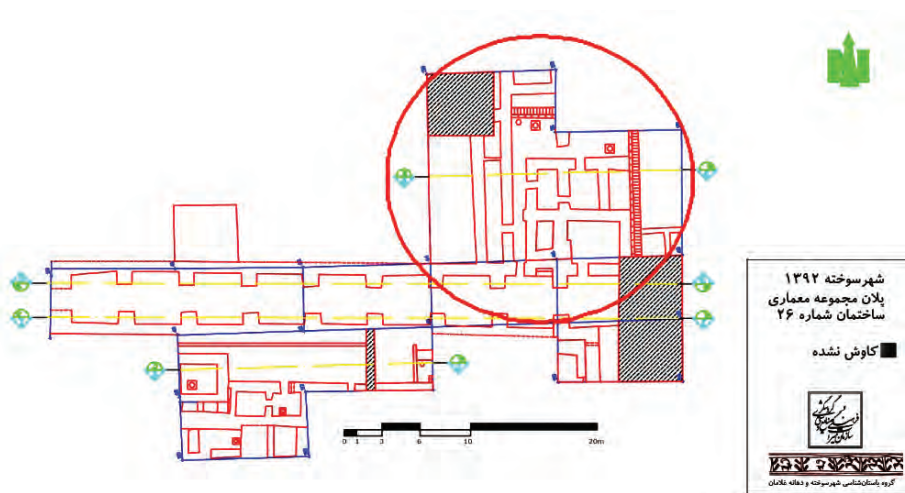
تصویر ۴۶. پلان ساختمان انباری
